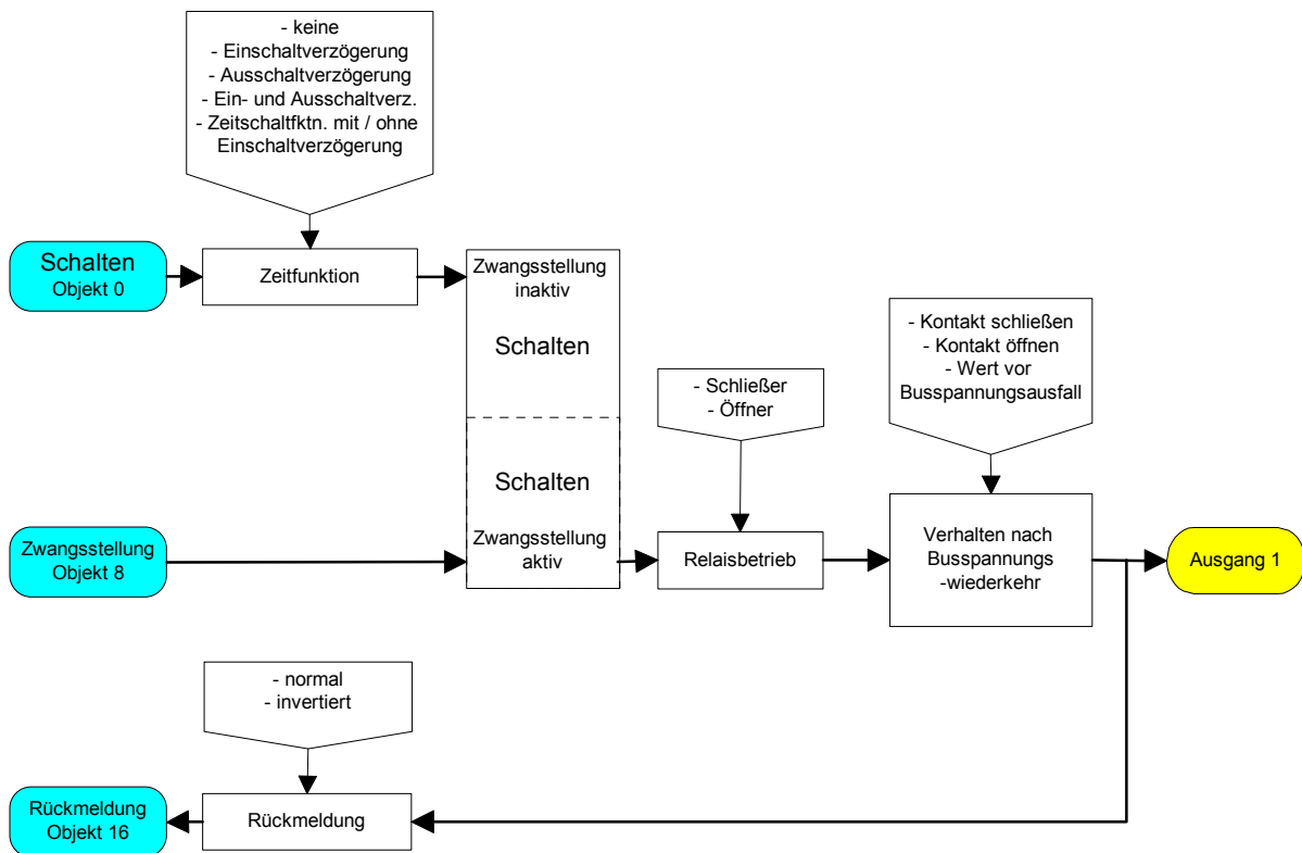
Funktionsschaltbild (für Schaltausgänge / z. B. Ausgang 1 mit der Zusatzfunktion "Zwangsstellungsobjekt")
