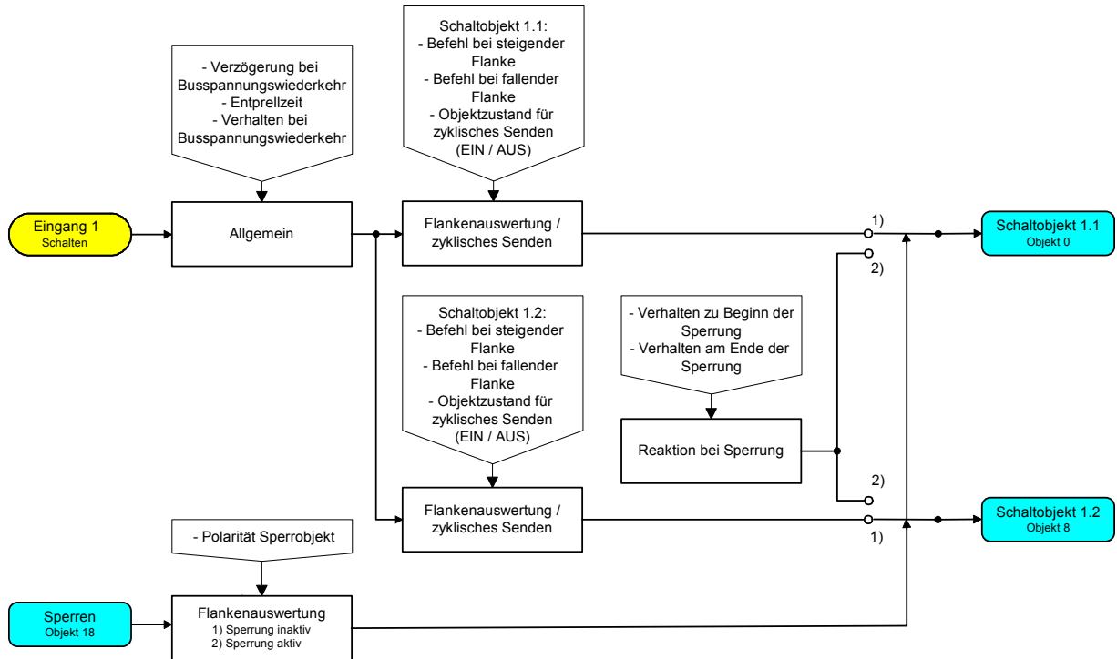
Funktionsschaltbild (für Binäreingang / z. B. Eingang 1 Funktion "Schalten")
